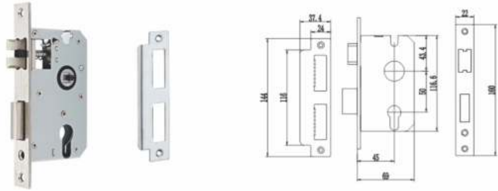
5002H-45 防插消音锁体
